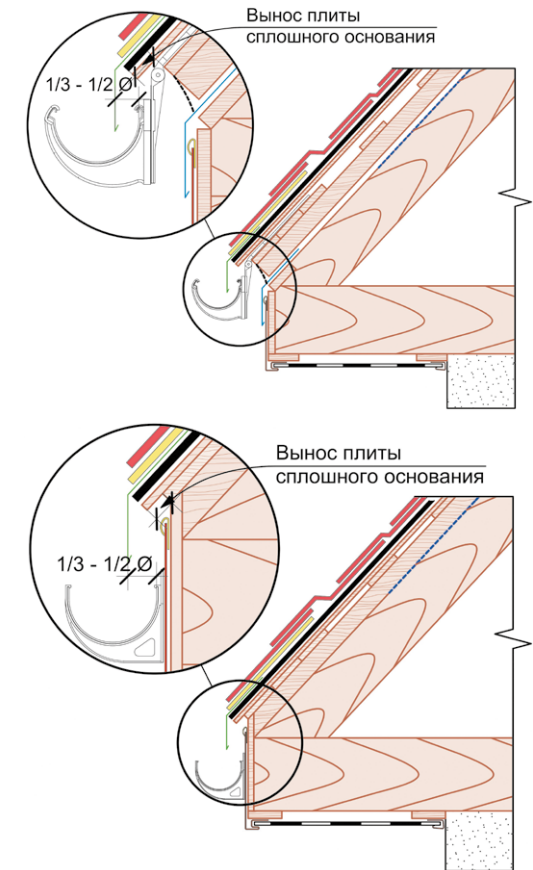
Рис. 6. Устройство выноса первого листа ОСП по отношению к первой доске обрешётки.
