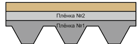
Рис. 19. Тыльная сторона гонта гибкой черепицы Döcke.
