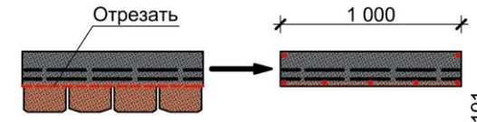
Рис. 18. Схема изготовления карнизной черепицы из рядовой и расположение гвоздей.
