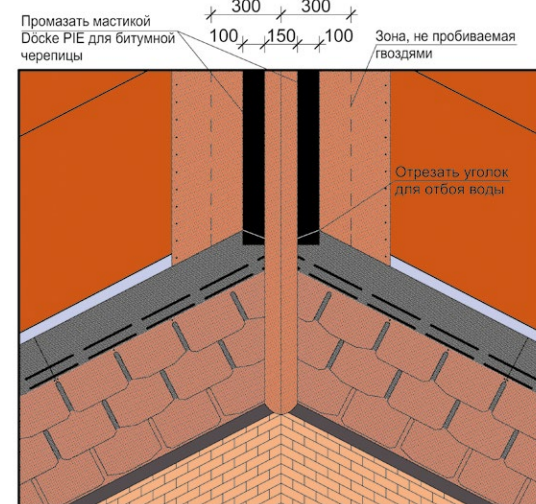
Рис. 27. Выполнение открытой ендовы.
