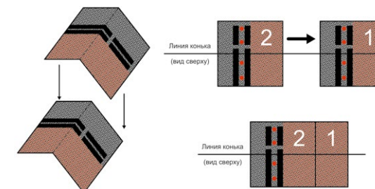
Рис. 33. Устройство рёбер скатов и коньков.
