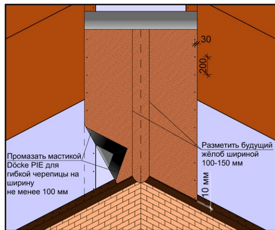
Рис. 14. Монтаж ендового ковра.
