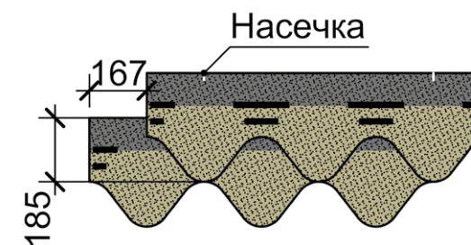
Рис. 24. Схема смещения гонтов по горизонтали и вертикали.
