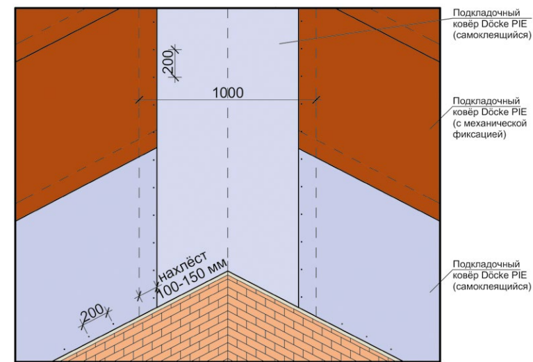
Рис. 12. Схема монтажа подкладочного ковора в ендове и на смежных скатах.
