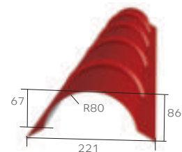
Планка конька круглого R80x2000 (Юг, Казахстан)
