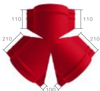
Y-образный тройник для круглого конька R110
