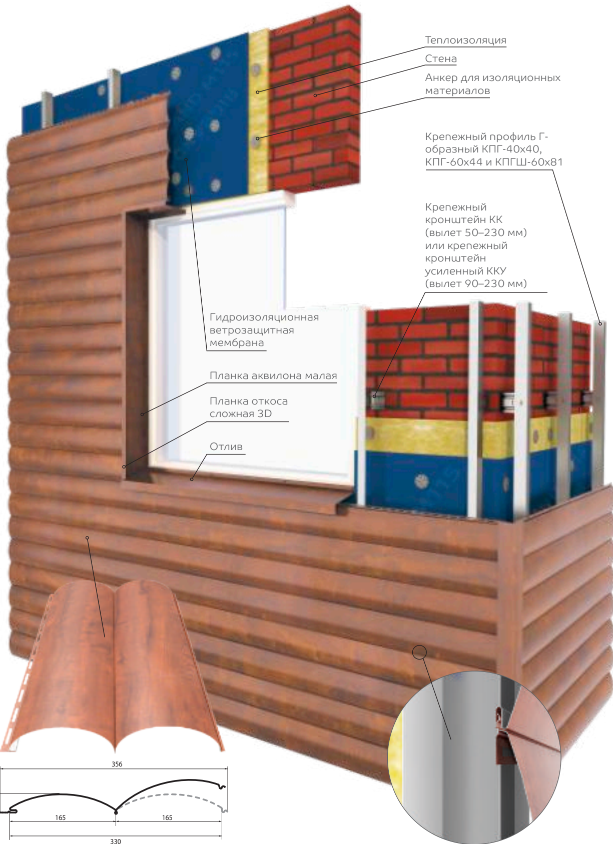
Стальной сайдинг Woodstock®-28x330 вид профилирования: гладкий
