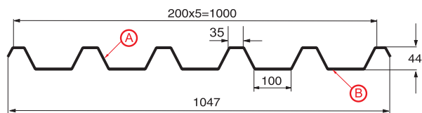
Профилированный лист С-44х1000-А Толщина материала: 0,45–0,8 мм
