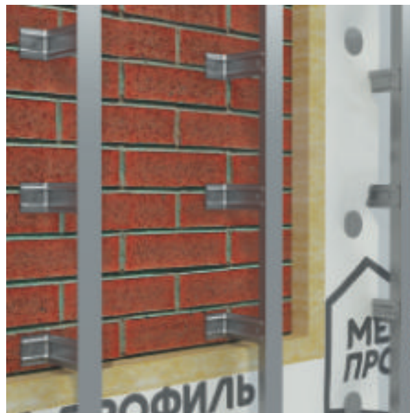
Крепежный профиль Г-образный КПГ-40x40x3000, t=0,9 мм
