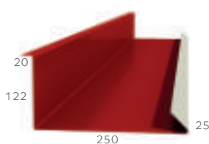
Планка примыкания нижняя 250x122x2000
