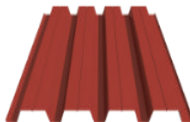
Профилированный лист МП-35x1035-B Толщина материала 0,45–0,9 мм
