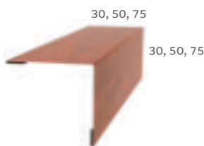
Планка угла наружного 30x30x3000, 50x50x3000 или 75x75x3000
