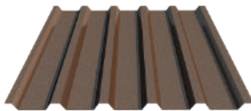
Профилированный лист C-21x1000-A Толщина материала 0,4–0,7 мм
