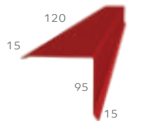
Планка торцевая 95x120x2000
