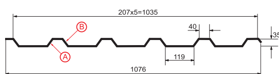
Профилированный лист МП-35x1035-B Толщина материала 0,45–0,9 мм
