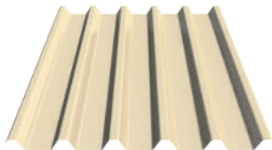
Профилированный лист НС-35х1000-В Толщина материала: 0,45–0,9 мм
